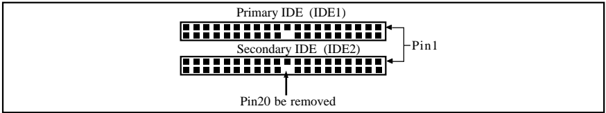
IDE Connectors
